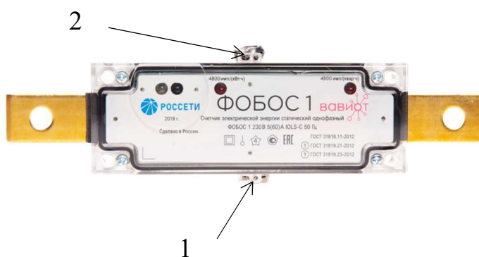
Счетчик исполнения «Сплит» «базовой» модели корпуса без клемных крышек
