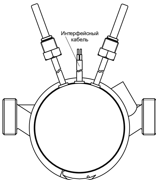
Рисунок 1. Расположение кабелей, проводных интерфейсов счетчиков тепла «Гефест», исполнений Гефест хх.хх.I, Гефест хх.хх.M, Гефест хх.хх.R и Гефест хх.хх.IF
