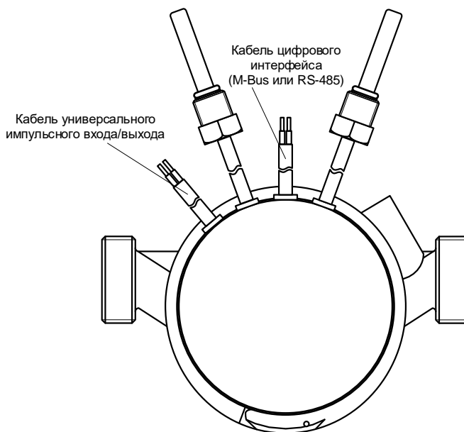
Рисунок 2. Расположение кабелей, проводных интерфейсов счетчиков тепла «Гефест», исполнений Гефест хх.хх.IM, Гефест хх.хх.IR
