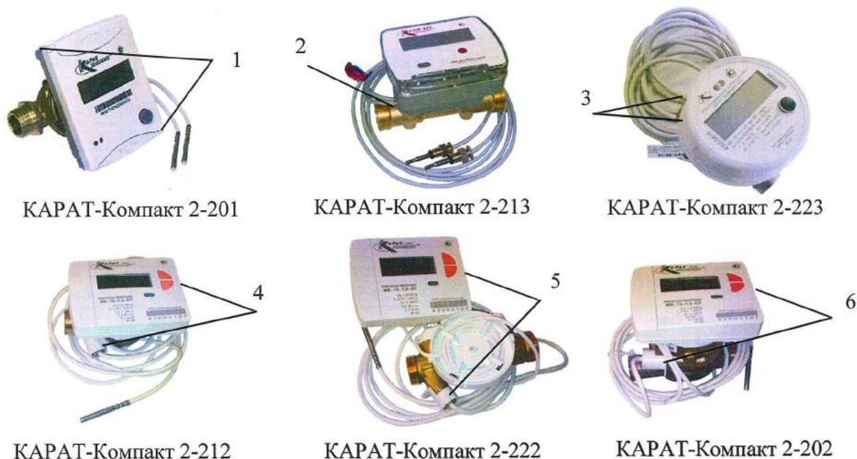
Рисунок 1 – Внешний вид теплосчетчиков КАРАТ-Компакт 2 и места их пломбирования
