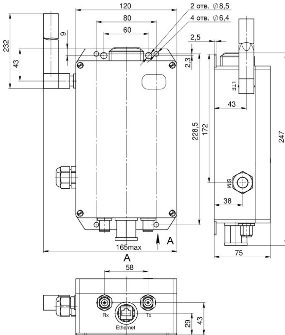
Рисунок А1 – Габаритные и установочные размеры блока приемо-передающего Базовой станции (GSM антенна показана условно).
