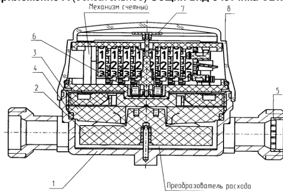
Приложение А (обязательное) Общий вид счетчика СВК
